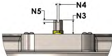
NAMUR TOP HAT DIMENSIONS
